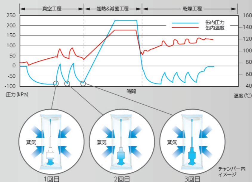
クラスBオートクレーブのイメージ
